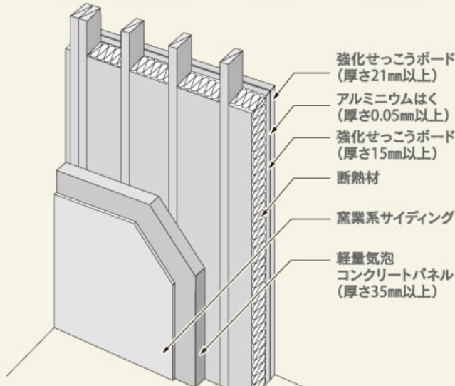
2×4工法に採用されている耐火性能をもつ外壁
