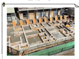
基礎工事
